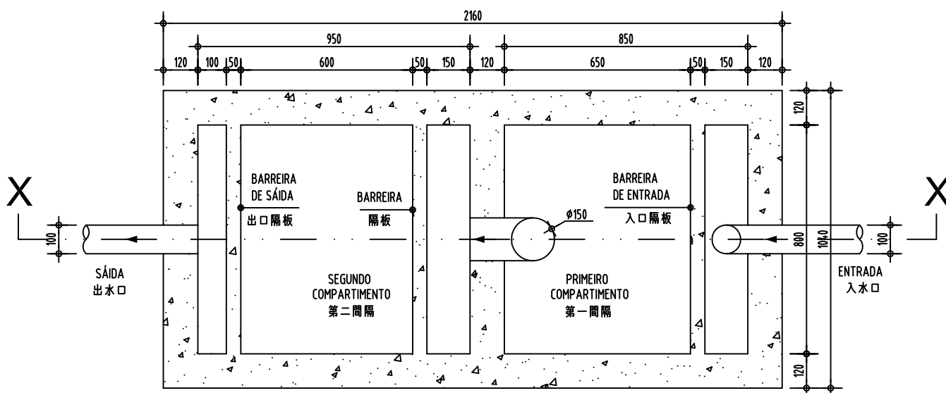
PLANTA 平面圖
