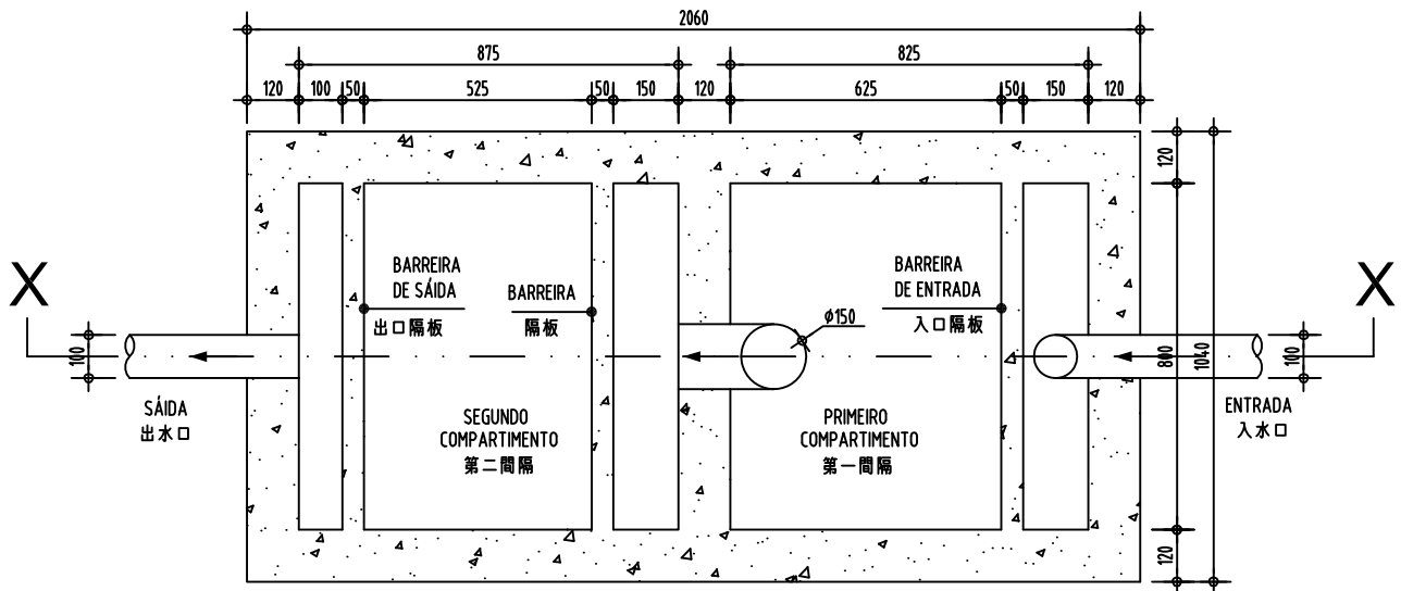
PLANTA 平面圖
