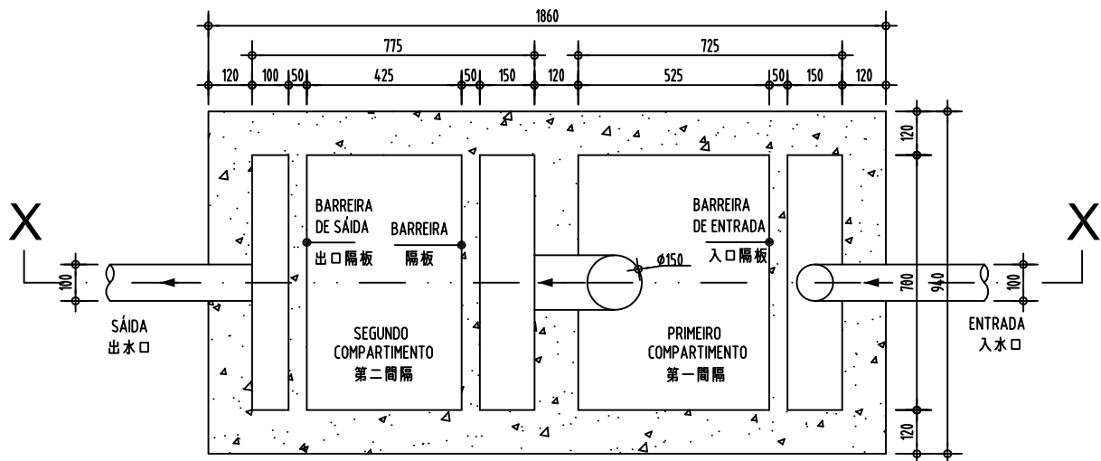
PLANTA 平面圖
