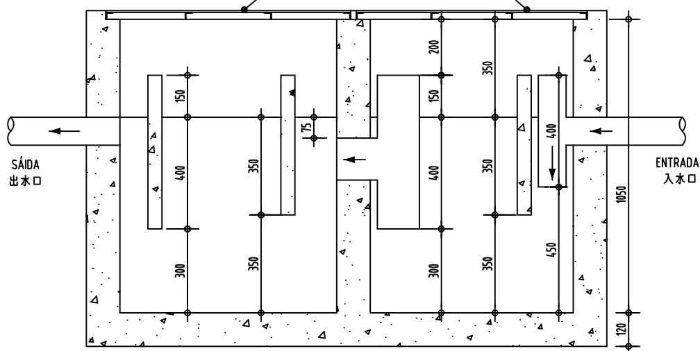
CORTE X-X 切面圖
