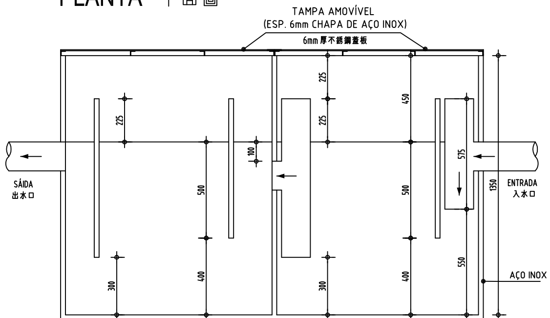
CORTE X-X 切面圖
