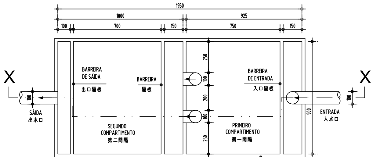
PLANTA 平面圖
