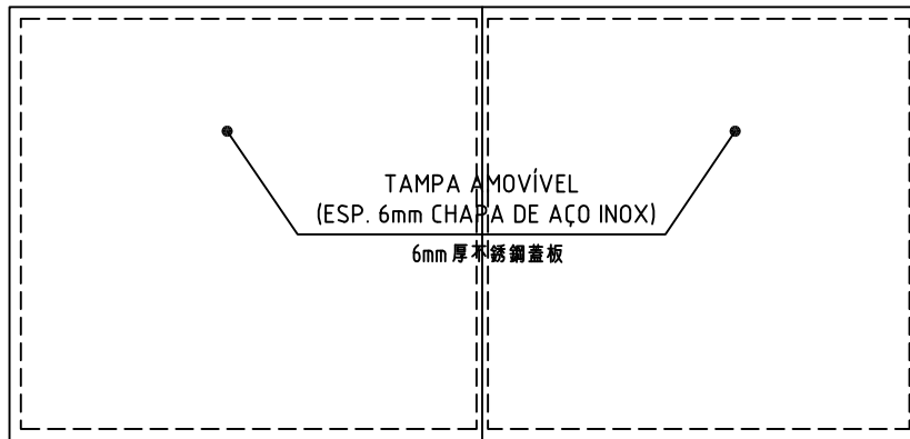
COBERTURA 頂視圖
