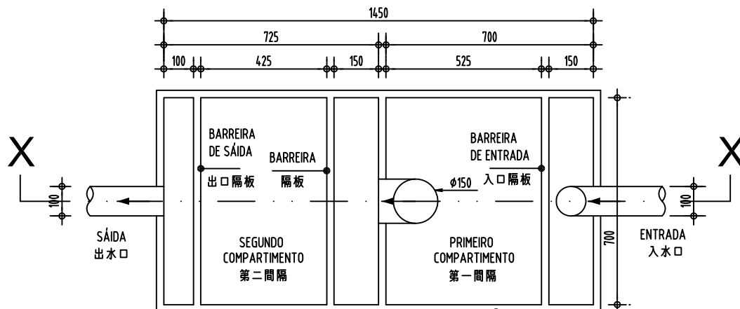
PLANTA 平面圖
