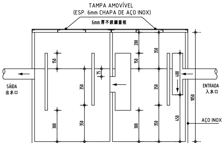
CORTE X-X 切面圖
