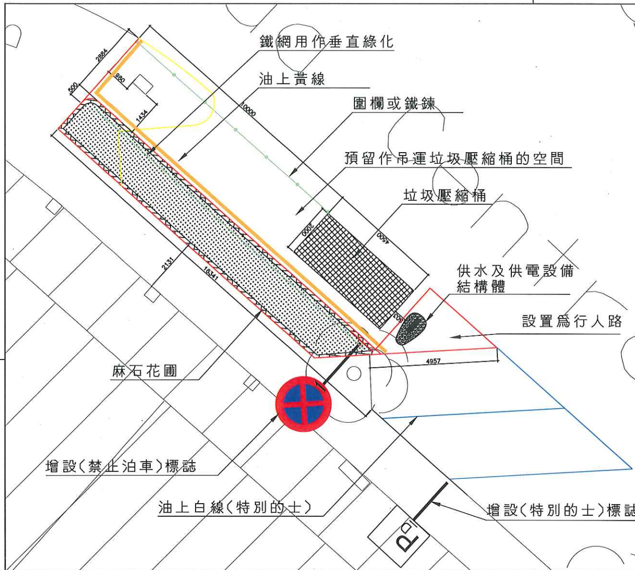
平面佈置圖 (1:100)
