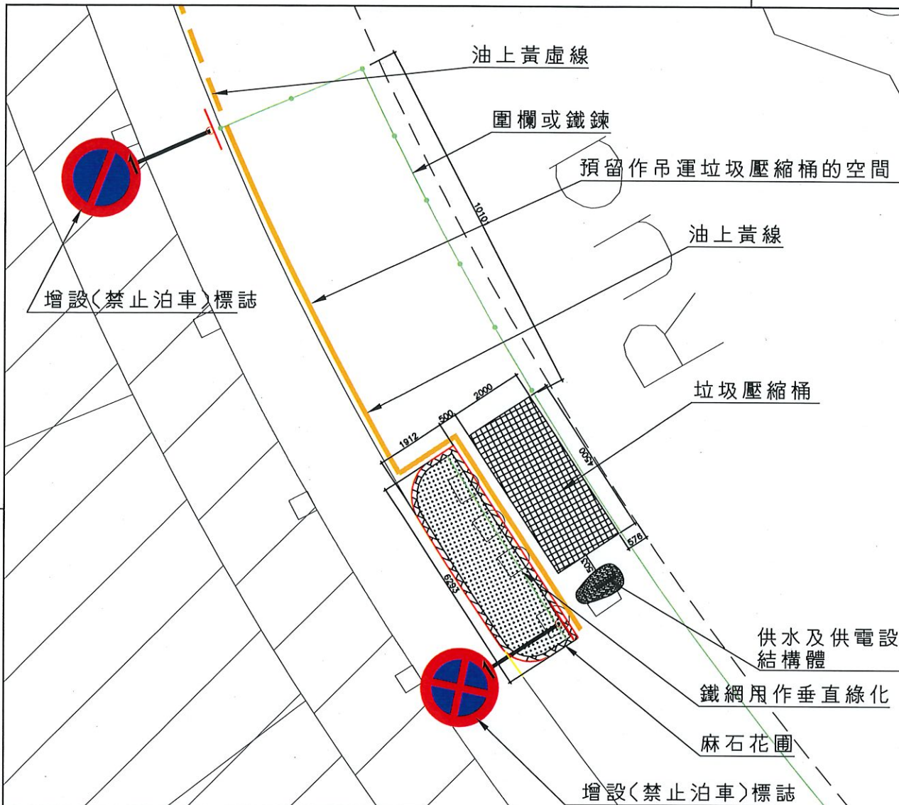
平面佈置圖 (1:100)
