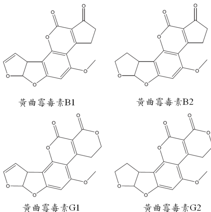
圖 1. 黃曲霉毒素 B1、B2、G1 和 G2 的結構圖
